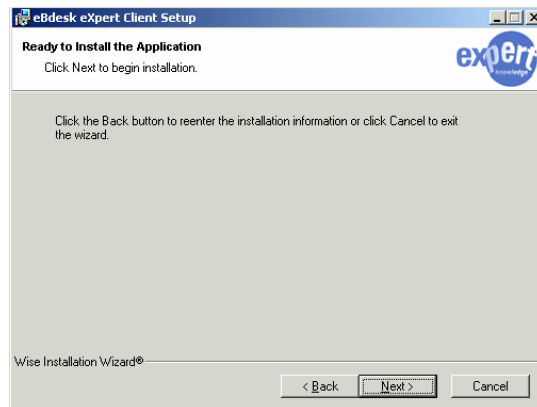
Gambar 1 - 5: Memulai Instalasi
